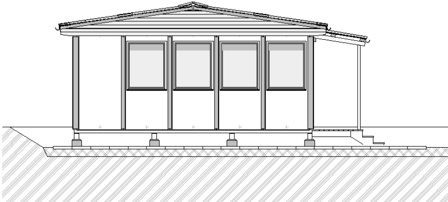
Fassade Süd-West
