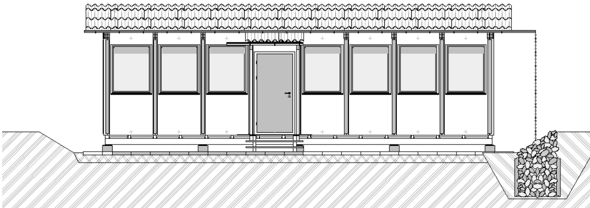
Fassade Süd-Ost
