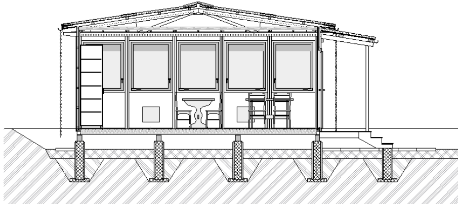
Querschnitt 1
