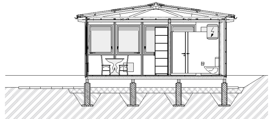
Querschnitt 2
