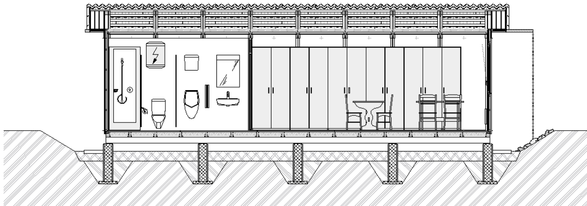
Längsschnitt 2
